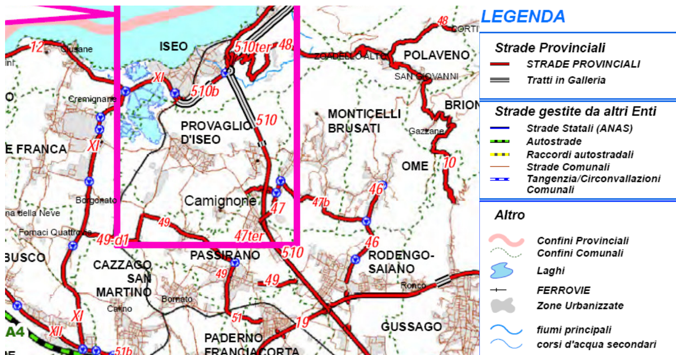
Classificazione amministrativa della rete stradale [Fonte: Piano del Traffico della Viabilità Extraurbana, 2012]
